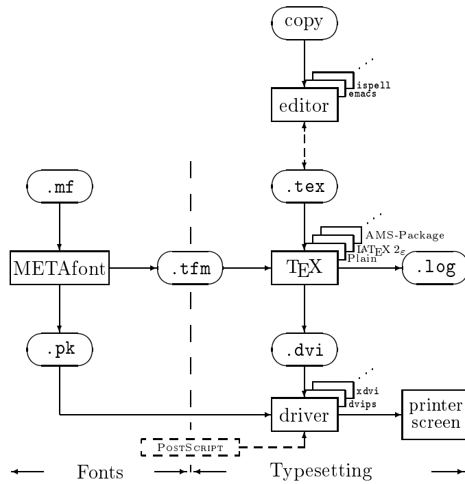
Рис. 1.1: Составляющее \text{T}_{\text{E}}\text{X} системы
